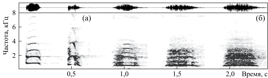
Рис. 1. Спектрограммы (внизу) и осциллограммы (вверху) двух криков тревоги индийского замбара (а) и трёх криков тревоги индийского мунтжака (б). Во втором крике замбара виден скачок основной частоты. В трёх криках мунтжака детерминированный хаос занимает соответственно 40, 80 и 100% длительности лаи.
